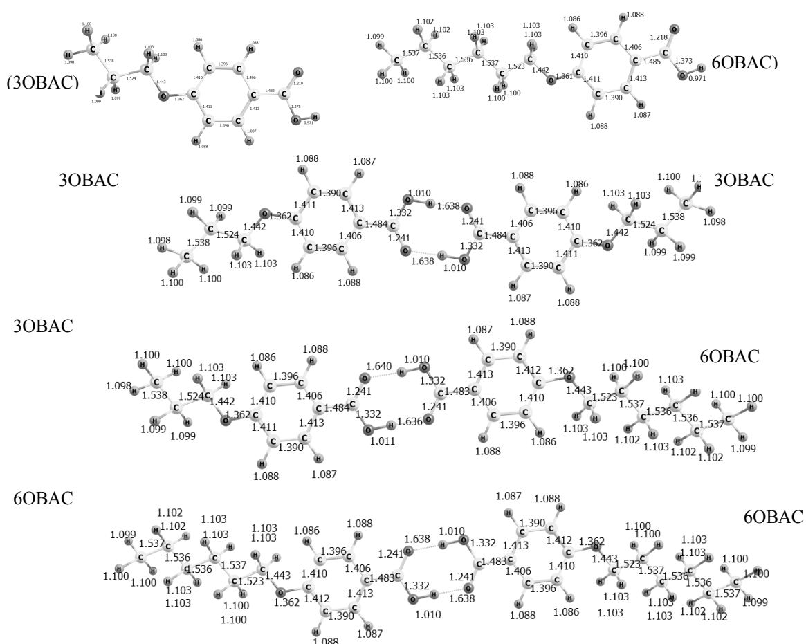
Рис. 1. Геометрическое строение и длины связей отдельных молекул и димерных Н-комплексов
