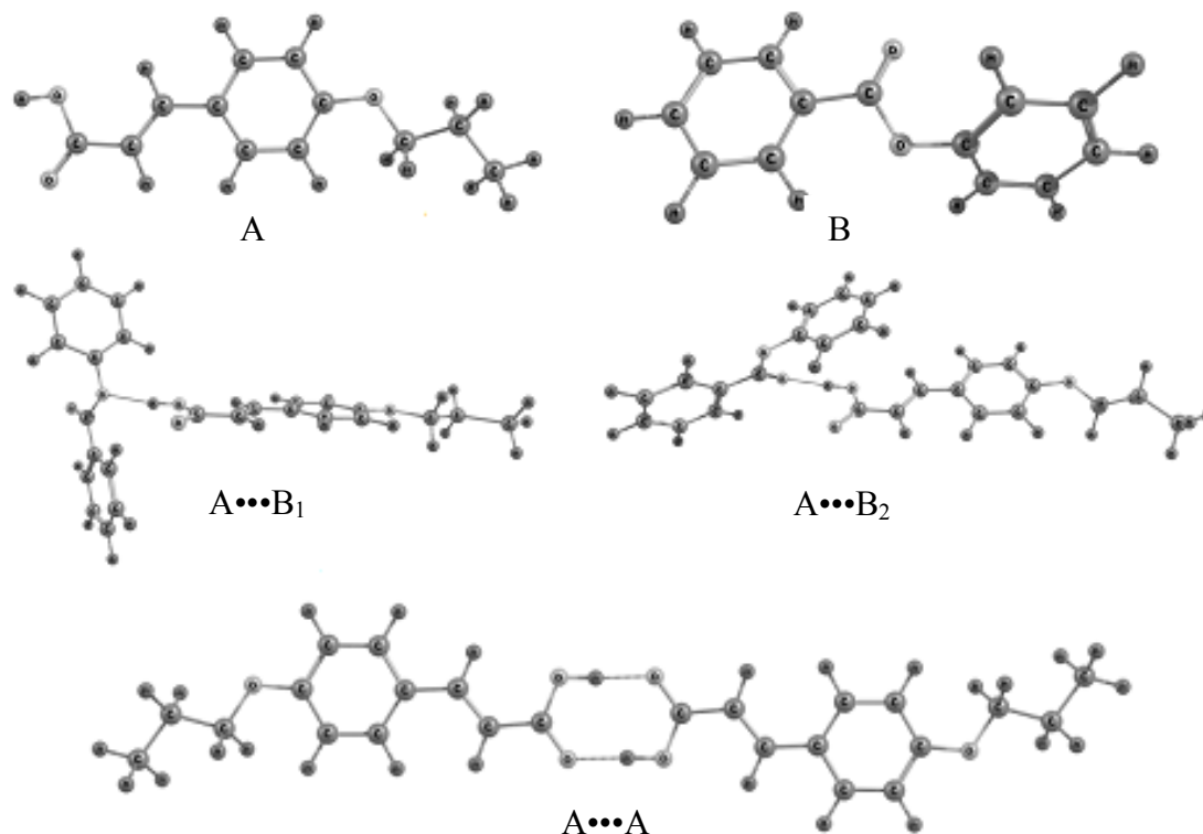
Рис. 1. Геометрическое строение исходных соединений и образующихся Н-комплексов
