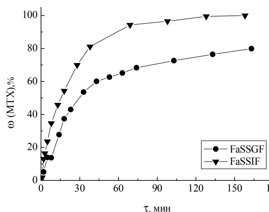
Рис. 2. Профили растворения метотрексата в биорелевантных средах
