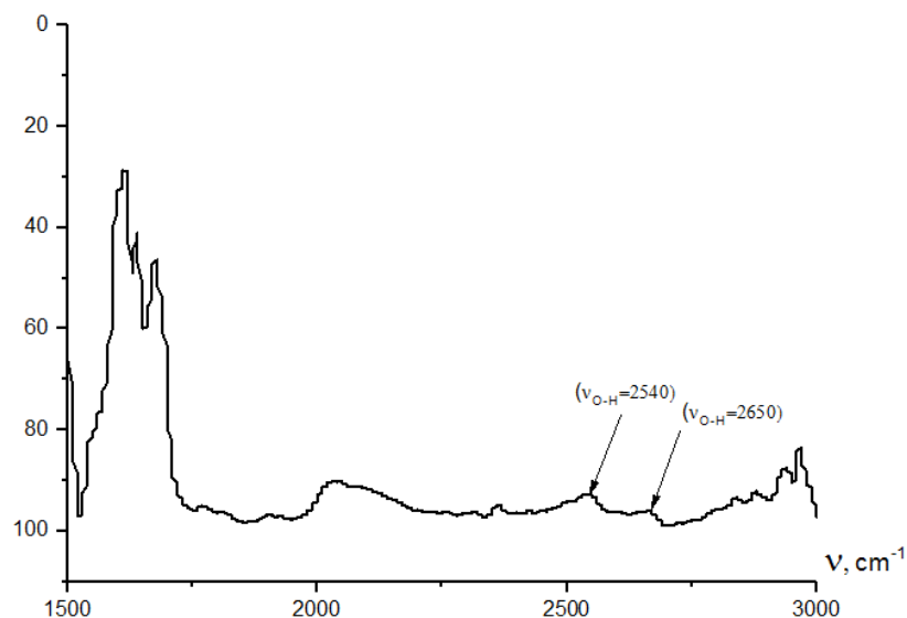
Рис. 2. Колебательный ИК-спектр системы А:В
