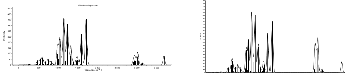
Рис. 2. ИКС мономерных молекул бензойных кислот
