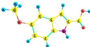
Рис. Геометрическое строение конформера молекулы 5-МИ-2-КК
