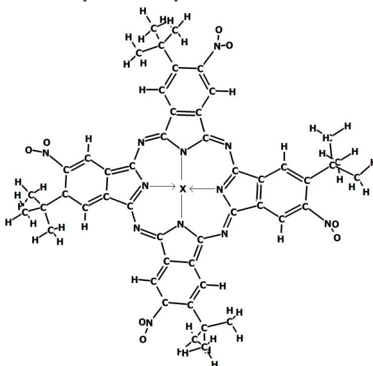
Рис. Строение металлокомплексов тетра-(4- трет -бутил-5-нитро)фталоцианина (X – Ni, Co)
