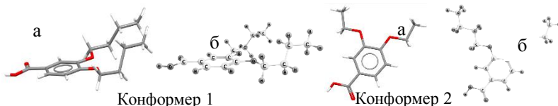
Рис. Строение 3,4 – диАОБК: 1а,2а – КБД, 1б,2б – B97D/6–311G**
