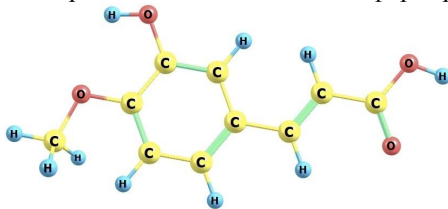
Рис. Геометрическое строение конформера молекулы 3-гидрокси-4-метоксикоричной кислоты
