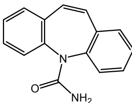
Рис. Структурная формула молекулы карбамазепина
