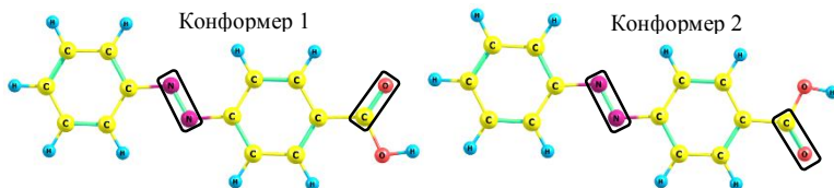
Рис. Геометрическое строение конформеров 4-ФАБК
