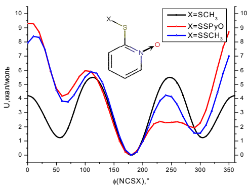
Потенциальная функция внутреннего вращения -\text{SX} вокруг связи \text{C}-\text{S}
