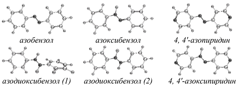
Рис. Оптимизированное геометрическое строение рассмотренных молекул
