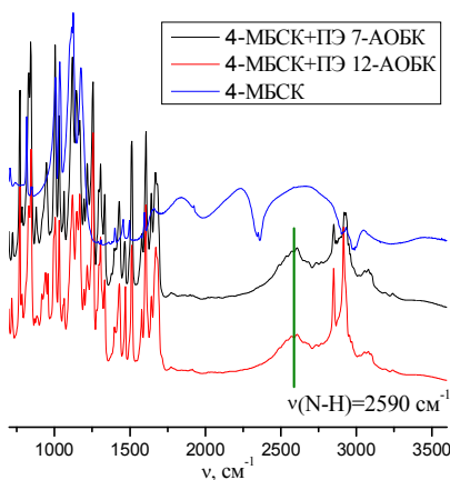
Рис. ИКС 4-МБСК и ее Н-комплексов
