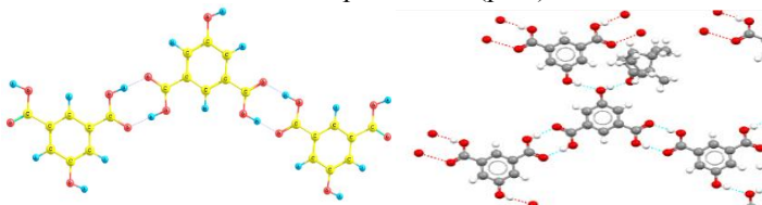
Рис. Структура Н-комплексов 5-ГИФК: а) расчет; б) КБД
