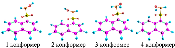
Рис. Геометрическое строение конформеров C_{10}H_9SO_3N
