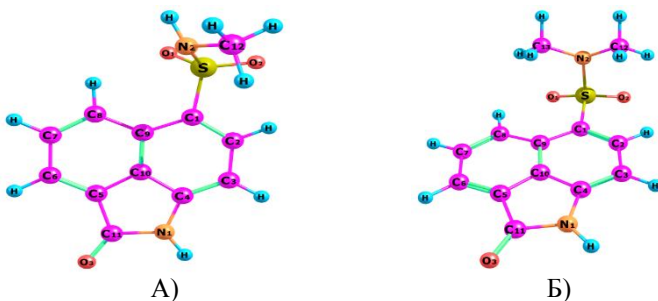
Рис. Геометрическое строение наиболее устойчивых конформеров исследуемых молекул
